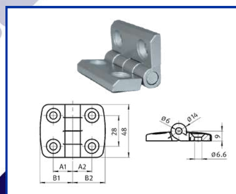
METALIC HINGE 30X30
